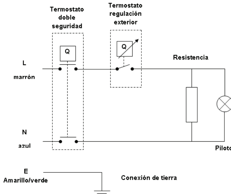
Fig. - 3 Esquema unifilar modelo APARICI - SB10
